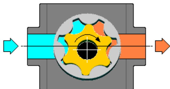
GEROTOR
