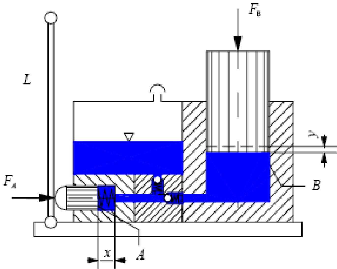
Hidraulički sistem-hidraulička dizalica
