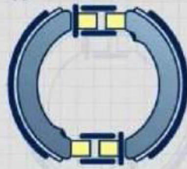
Duo-dupleks
