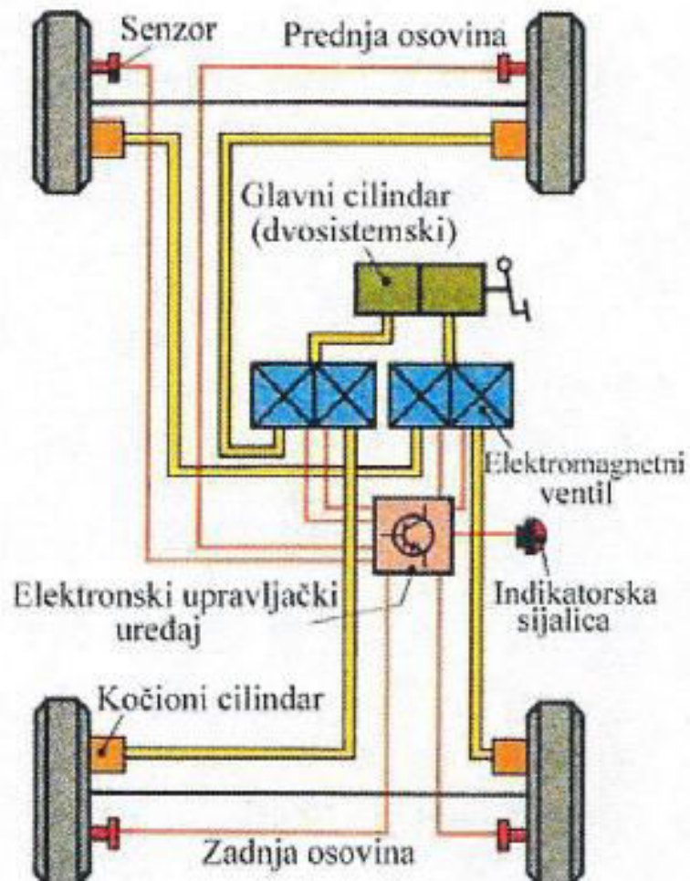
četvorokanalni sistem
