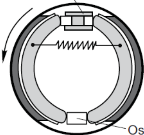
SIMPLEX KOČNICA
