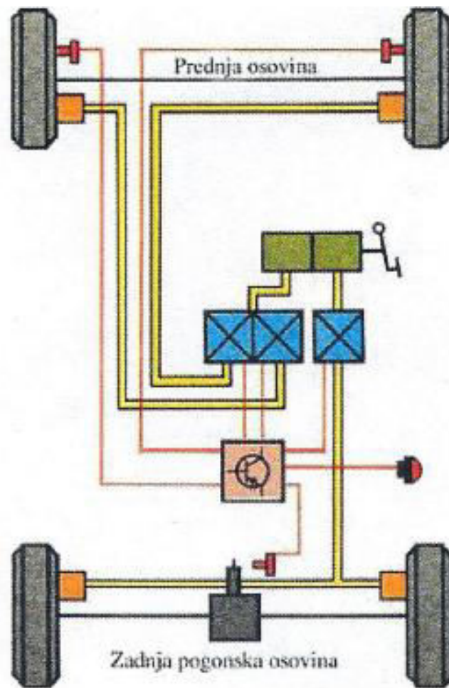
trokanalni sistem
