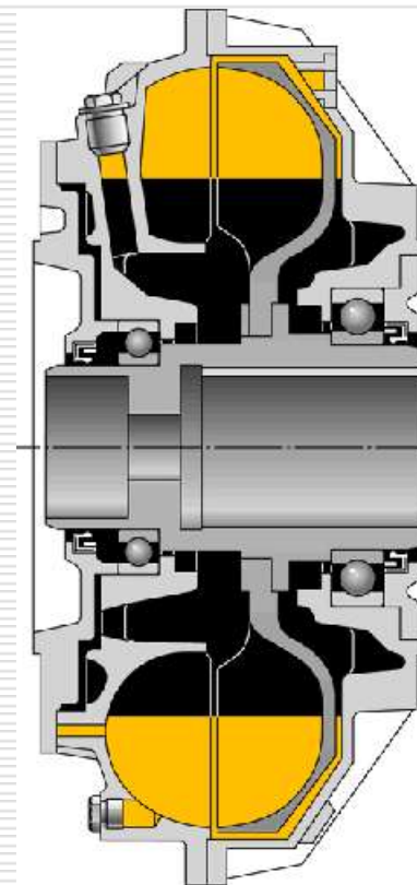
Радни режим
