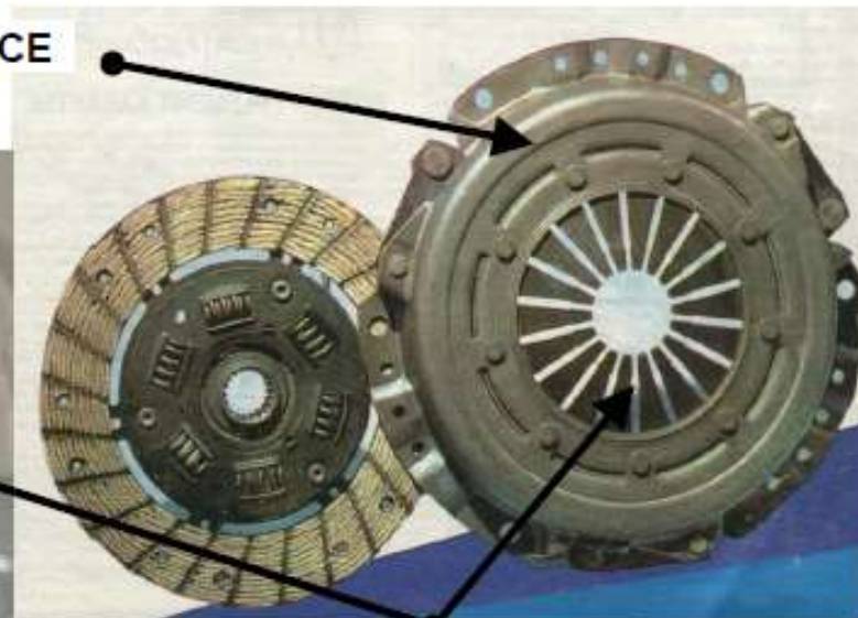
TANJIRASTA OPRUGA
