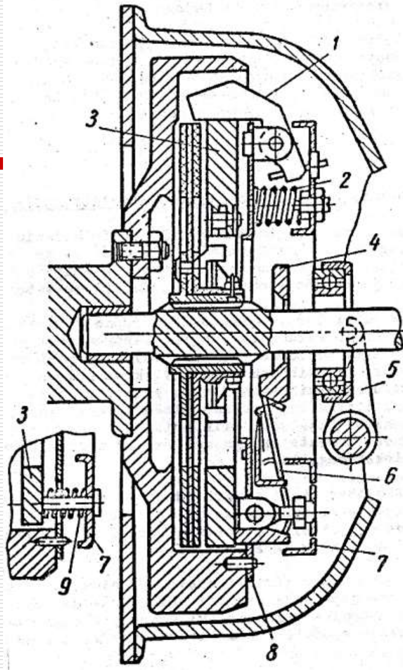
Центрифугална спојница
