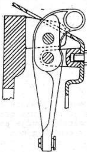
Полуцентрифугална спојница
