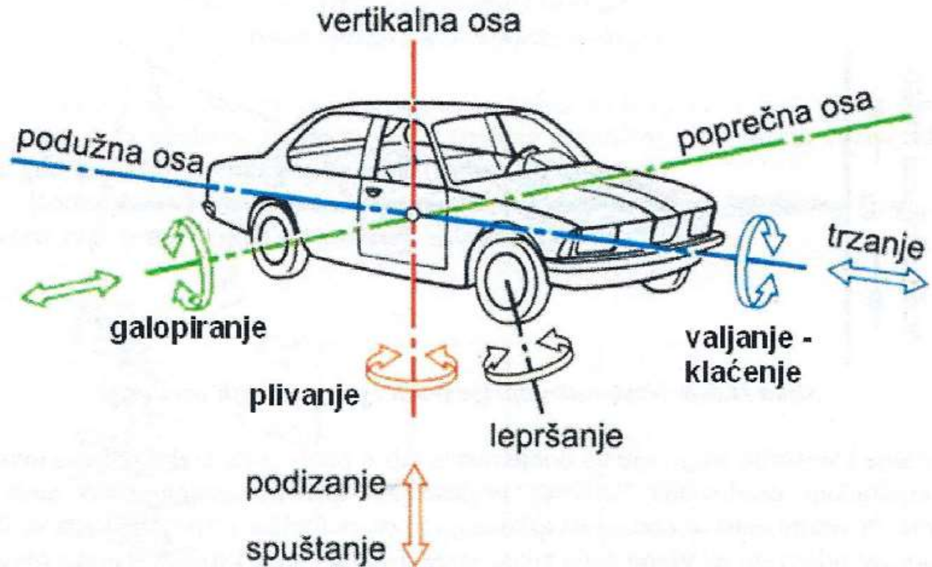
Приказ претпостављених и предвиђених кретања маса возила
