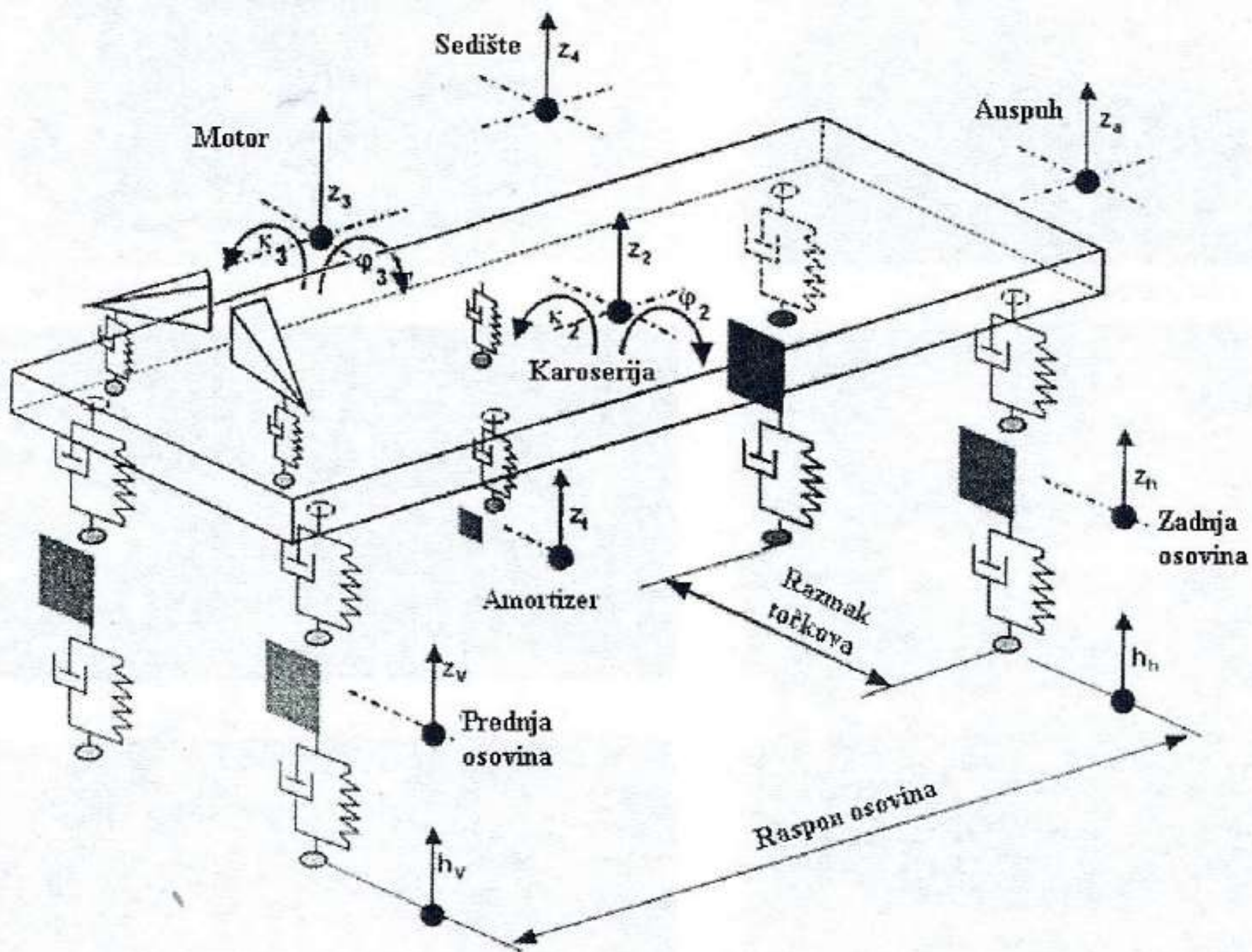
Осцилаторни модел друмског возила
