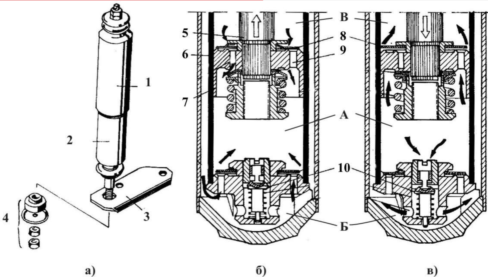
Амортизер (телескопски)
