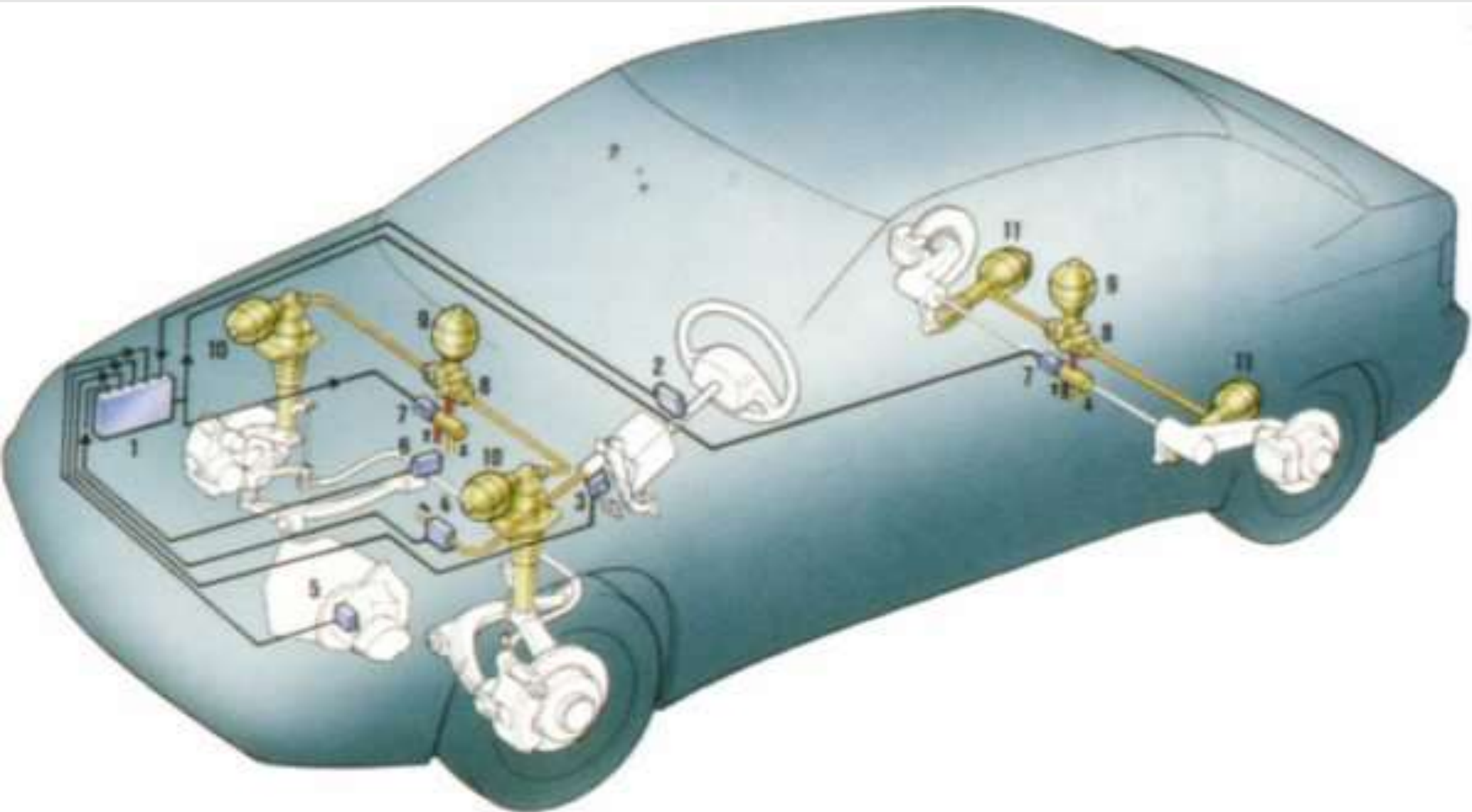
Активни систем ослањања Hydractive III, фирме Citoren
