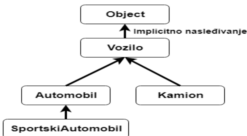
Slika 2.1 – Dijagram zavisnosti klasa
