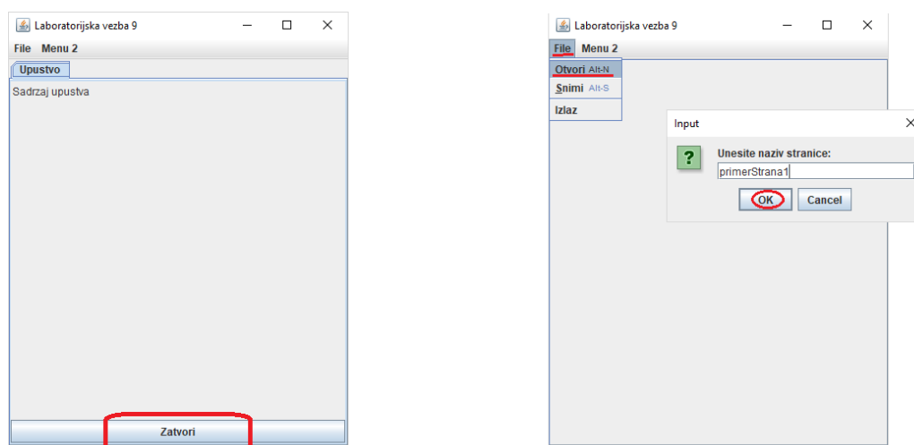
Slika 9.3- Zatvaranje stranice pane-a, dijalog za unos
