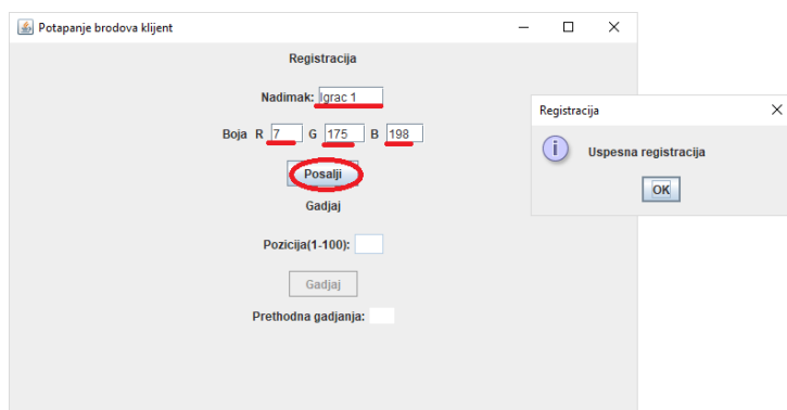
Slika 10.5- Registracija korisnika
