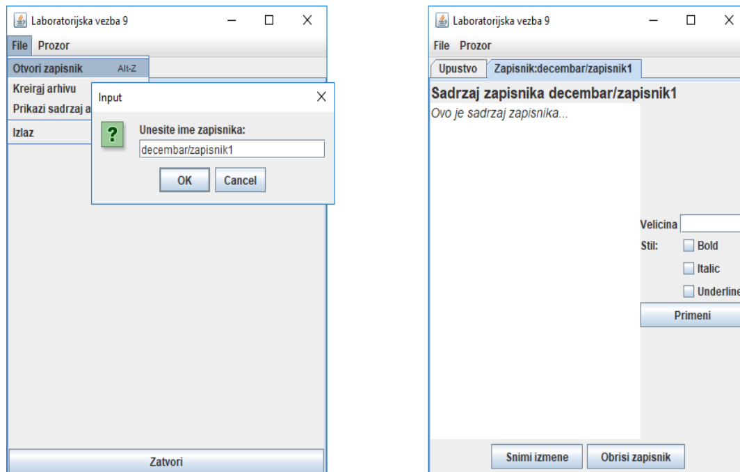
Slika 9.6- Otvaranje/kreiranje zapisnika
