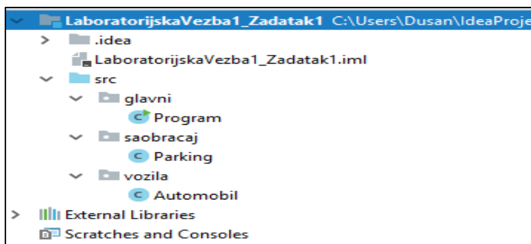
Slika 2.2- Struktura projekta
