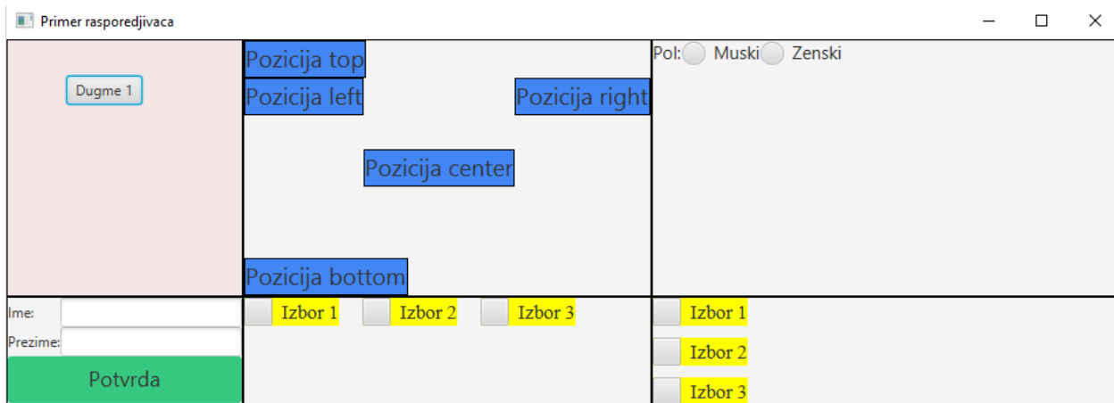
Slika 12.3- Raspoređivači
