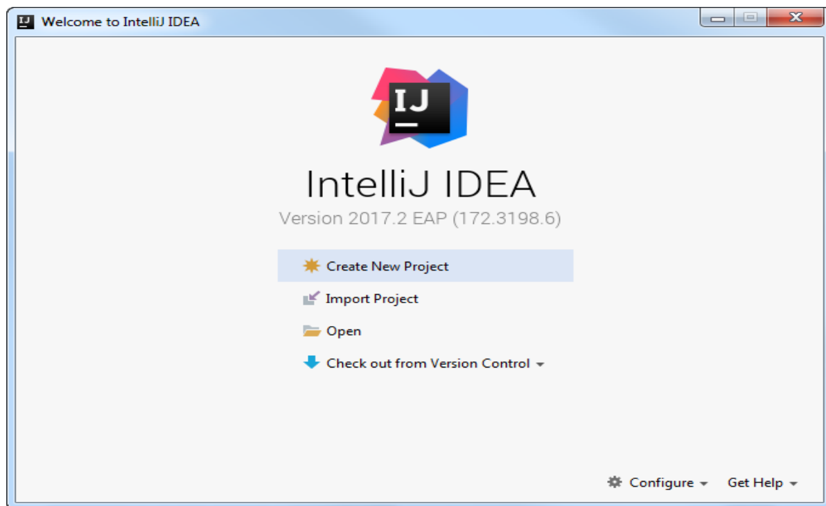
Slika 1.5- Kreiranje/otvaranje projekta
