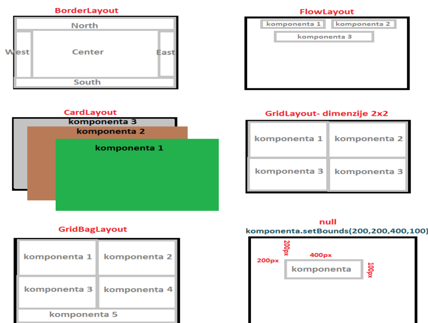
Slika 7.2- Raspoređivači
