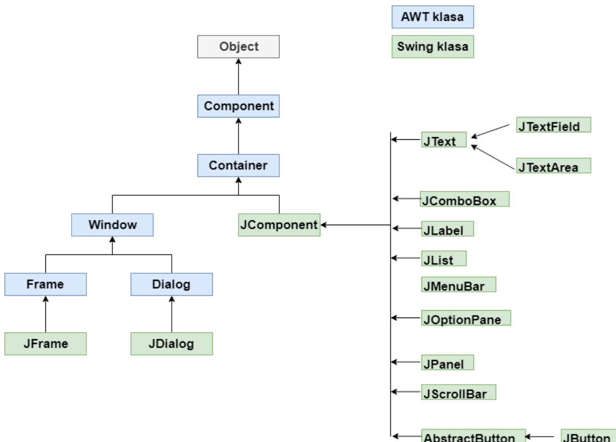
Slika 9.1- Hijerarhija bitnijih klasa
