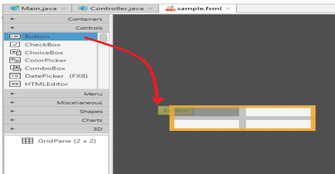
Slika 12.6- Dodavanje komponente (Button- a) prevlačenjem
