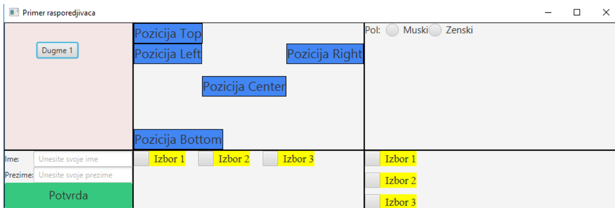
Slika 11.6 - Raspoređivači
