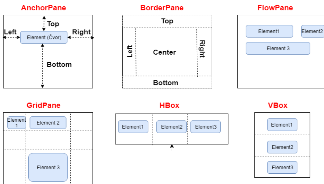
Slika 11.5 – Okviri rasporeda
