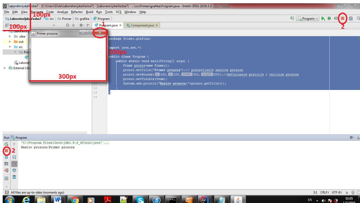
Slika 7.2- Glavni prozor
