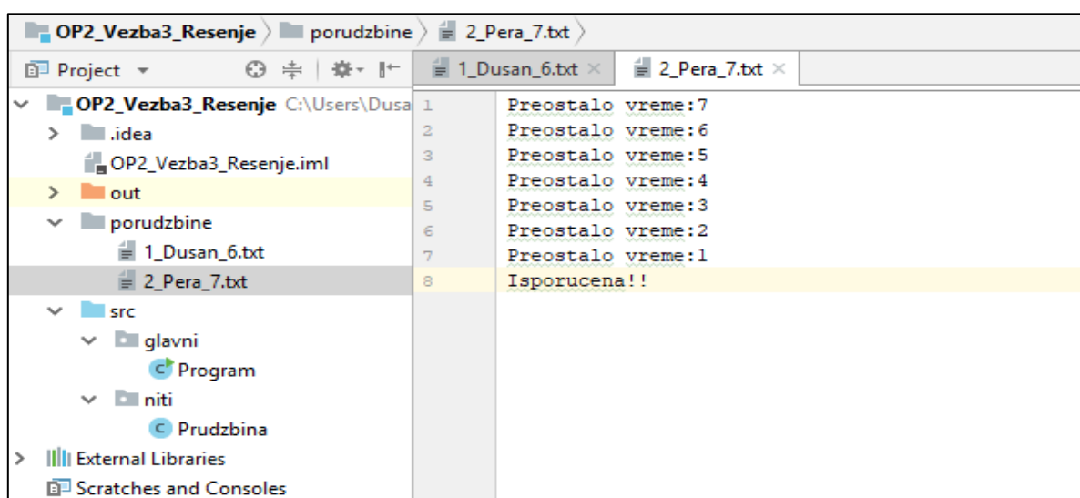
Slika 5.2- Rezultat izvršenja
