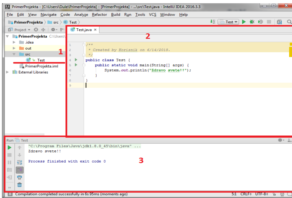
Slika 1.10- Testiranje okruženja
