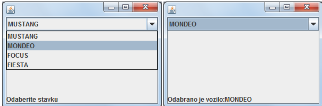
Slika 5.46. Izgled aplikacije PrimerJComboBox
