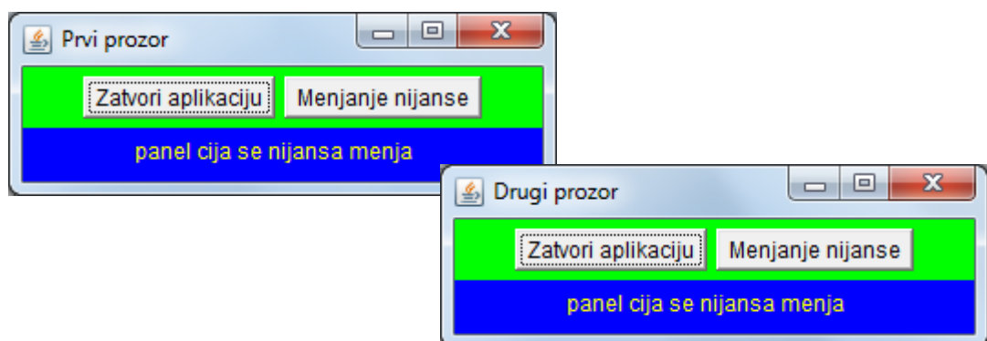
Slika 5.19. Izgled dve instance panela koji sadrži dva panela
