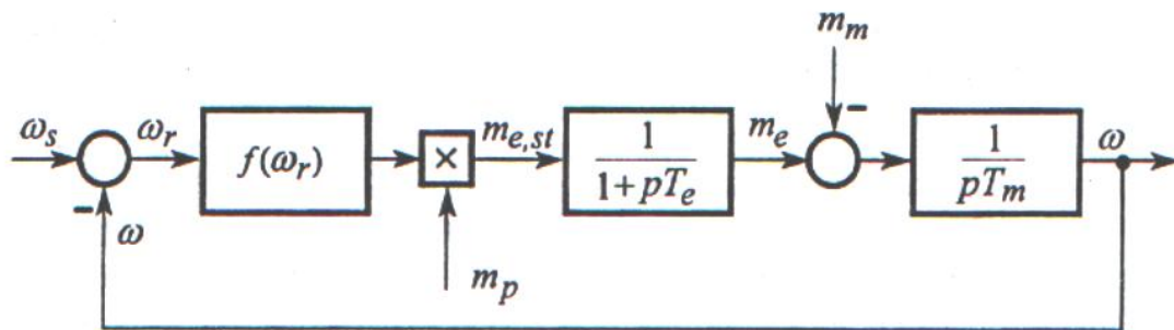
Sl. 5.4. Dinamička blok-šema asinhronog motor drugog reda prilagođena za analize regulacionih sistema
