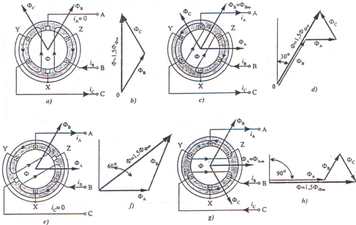
Sl. 3.3 Smerovi struja u namotajima statora i magnetni fluksovi u unutrašnjosti mašine (a,c,e,g) i ukupni magnetni fluks (b, d, f, h); a, b – za t=0 ; c, d – za t_1=T/12 ; e, f- za t_2=T/6 ; g, h – za t_3=T/4
