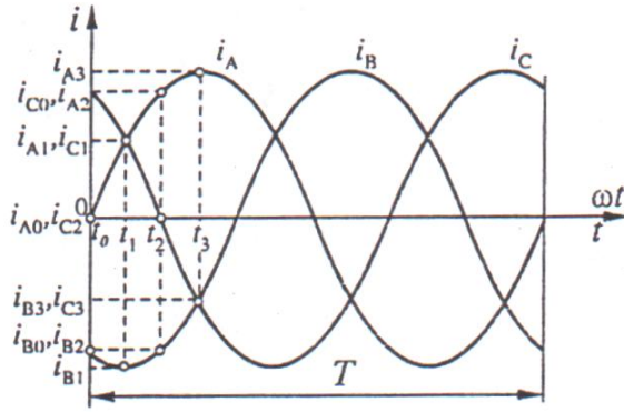
Sl. 3.2 Vremenska promena struje u faznim namotajima
