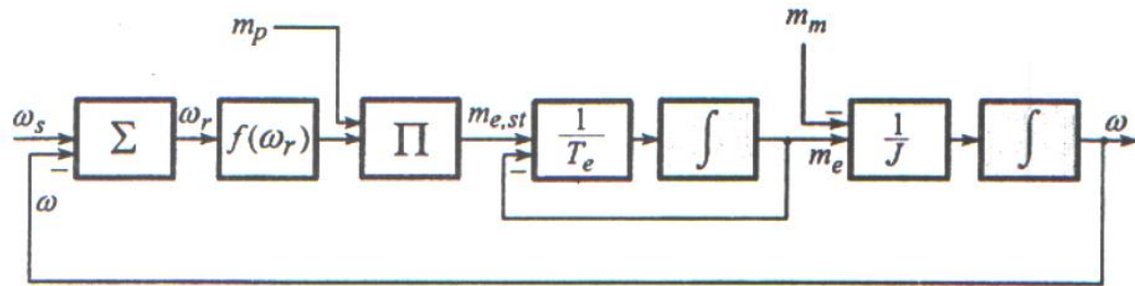
Sl. 5.3. Dinamička blok-šema asinhronog motor drugog reda
