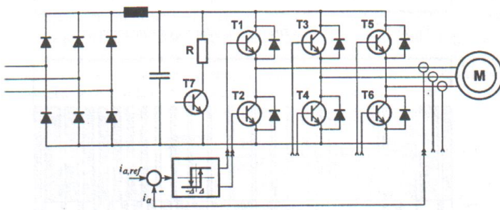
Sl. 5.7. Pogon sa struno regulisanim tranzistorskim invertorom
