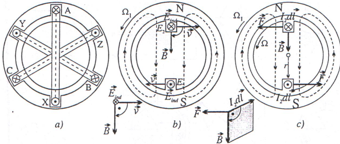
Sl. 3.4 Principijelna šema rada asinhronog motora
