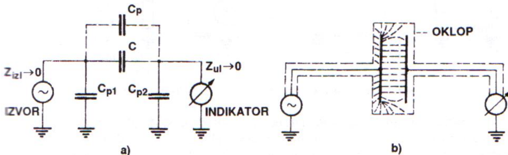
Slika 10.7. Priključivanje kapacitivnog senzora: a) potencijalno-strujna šema, b) elektrostatika zaštita
