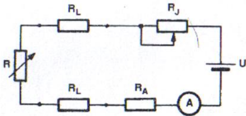
Slika 9.3. Distanciono merenje otpora I-metodom
