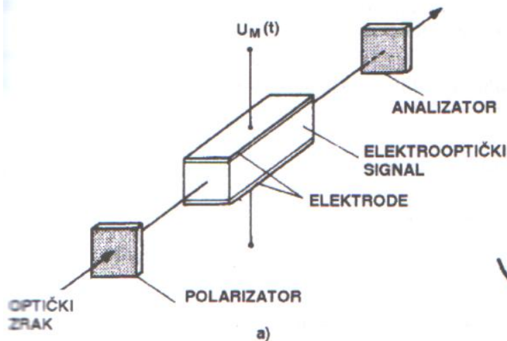
Modulacija na bazi elektrooptičkog efekta: a) Kerova ćelija, b) modulaciona karakteristika
