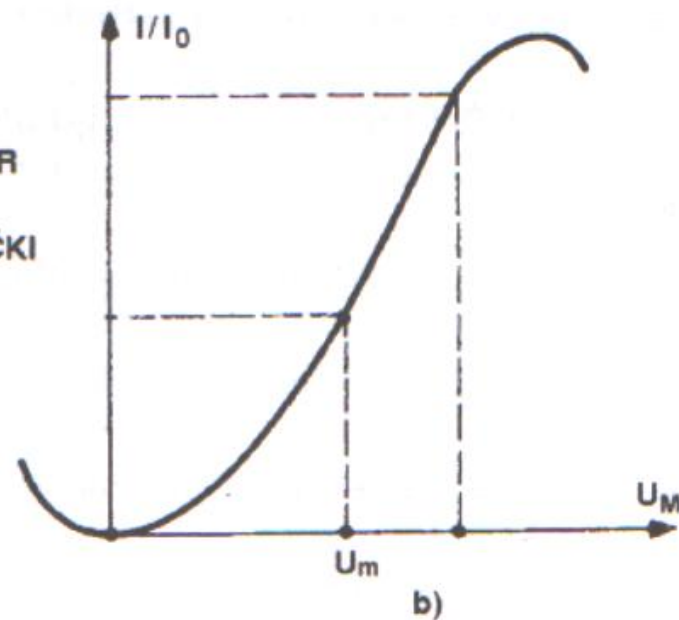
Modulacija na bazi elektrooptičkog efekta: a) Kerova ćelija, b) modulaciona karakteristika
