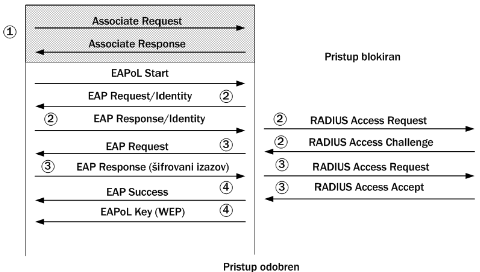
Slika 9.25. EAP autentifikacija
