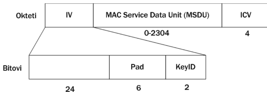
Slika 9.12. WEP okvir
