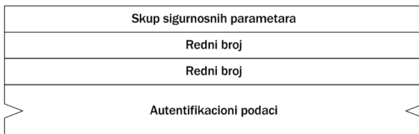
Slika 4.6. AH zaglavlje
