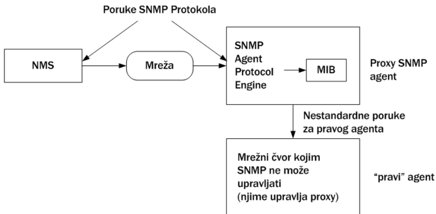
Slika 11.7. Proxy agent
