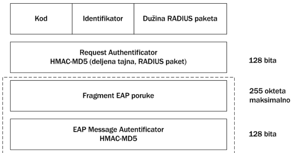
Slika 9.26. RADIUS paket
