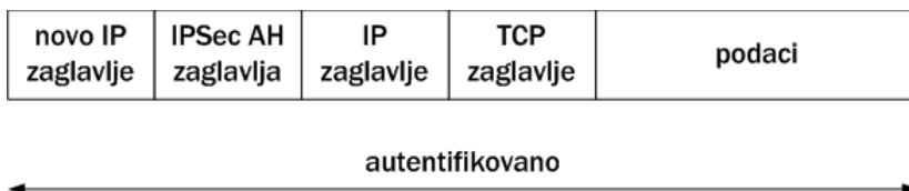
Slika 4.13. AH tuneliranje
