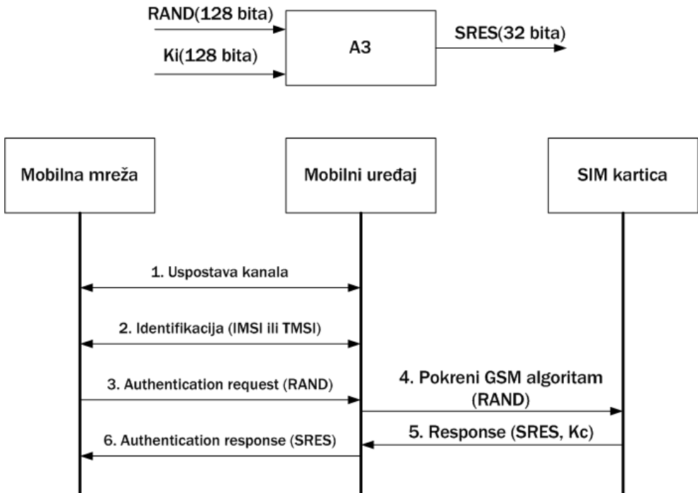
Slika 9.33. Proces autentifikacije
