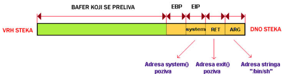
Slika 10.2. Izgled steka prilikom iskorišćavanja propusta ret-into-libc tehnikom
