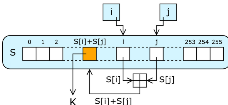
Slika 9.14. RC4
