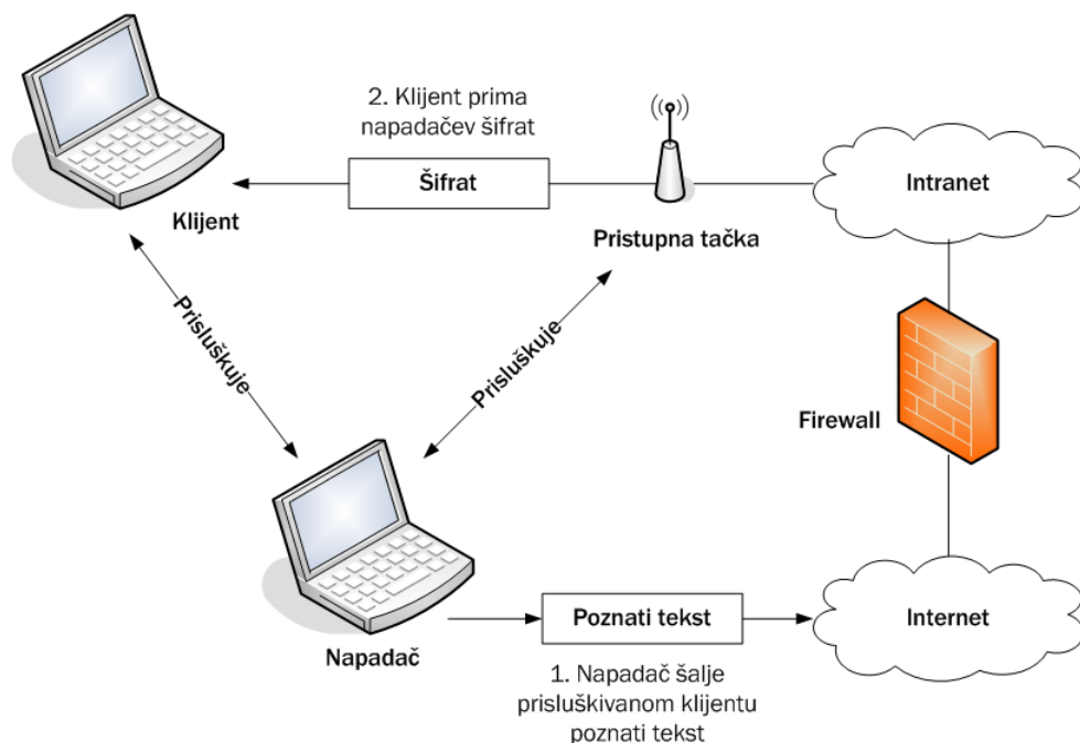
Slika 9.15. Napad ponavljanjem inicijalizacionog vektora
