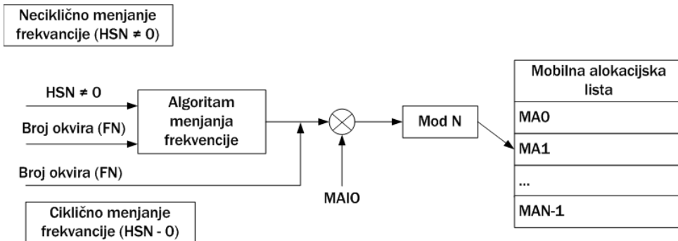
Slika 9.39. Promena frekvencije
