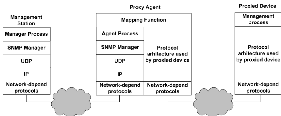
Slika 11.8. SNMP proxy
