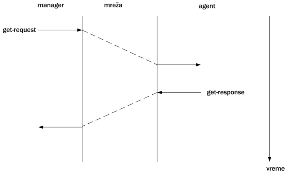
Slika 11.5. Manager / Agent model (get request operacija)
