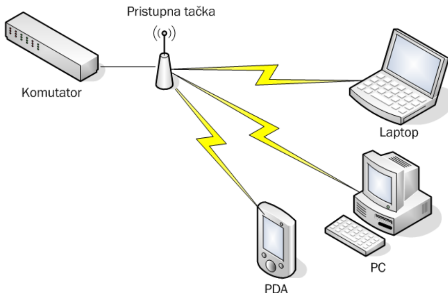
Slika 9.3. Pristupna tačka
