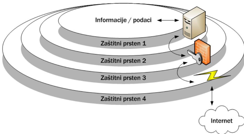
Slika 1.10. Slojevita zaštita
