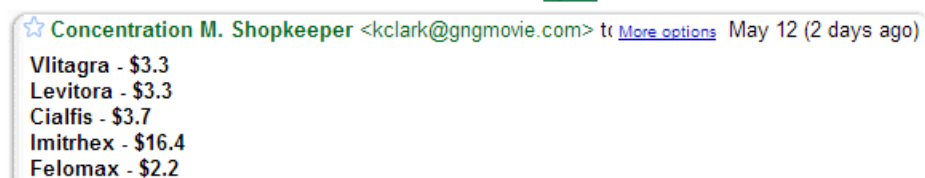
Slika 8.3. Primer SPAMa
