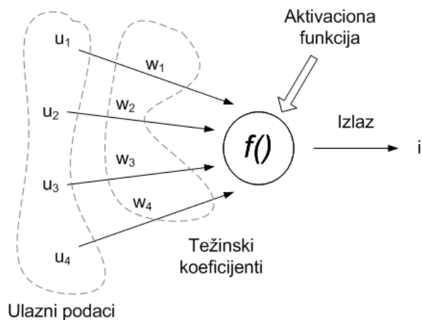
Slika 6.7. Model neurona
