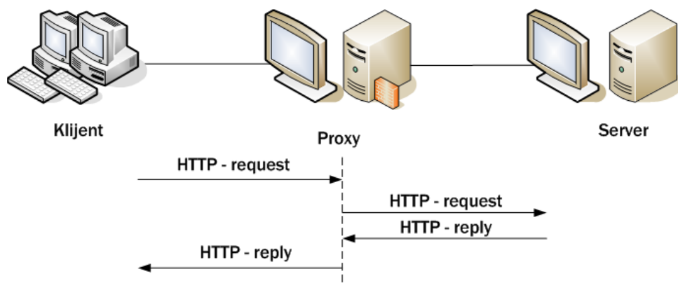
Slika 5.5. HTTP proksi
