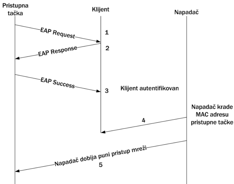
Slika 9.27. Krađa sesije
