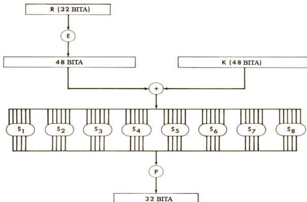
Slika 2. Jedna runda DES algoritma
