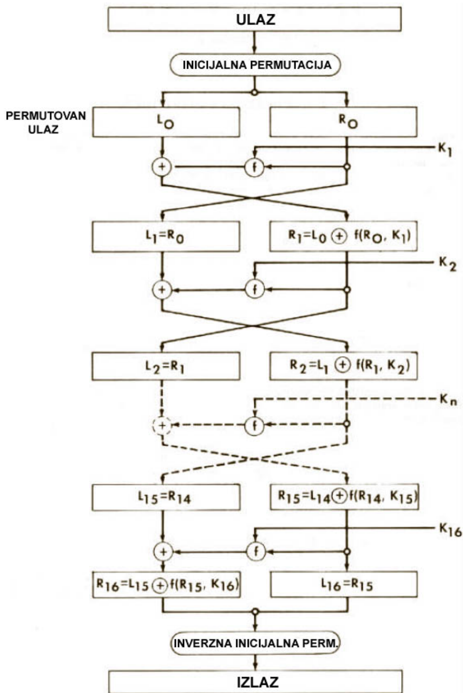
Slika 4. DES algoritam
