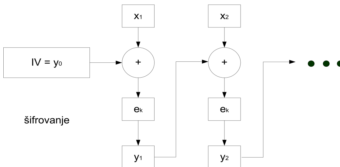
Slika 5. CFB režim
